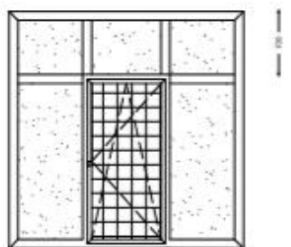
1. Ferestre parter, etajul N1; 1700-x2280(h) -32buc
