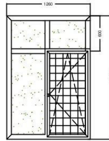
1. Ferestre ; 1260-x1760(h) -1buc
