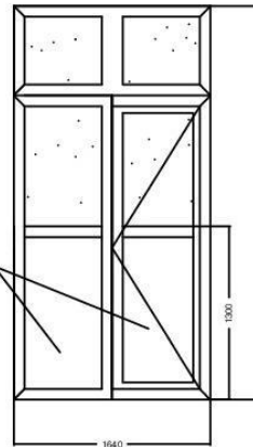
Usi intrare camin 1640x2280(h) -1 buc
