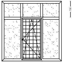
1. Ferestre parter, etajul N1; 1700-x2280(h) -32buc
