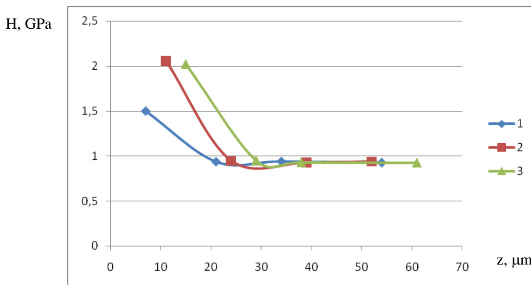
Fig. 3.15. Dependența microduranței de adâncimea stratului superficial pentru oțel aliat cu electrod - sculă din R6M5, timpul de prelucrare t=3\text{min/cm}^2 , 1) regim fin de prelucrare 2) regim mediu de prelucrare, 3) regim dur de prelucrare [20].
